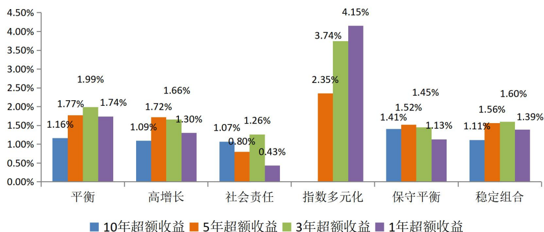
图 5 super/TTR 账户各组合超额收益
