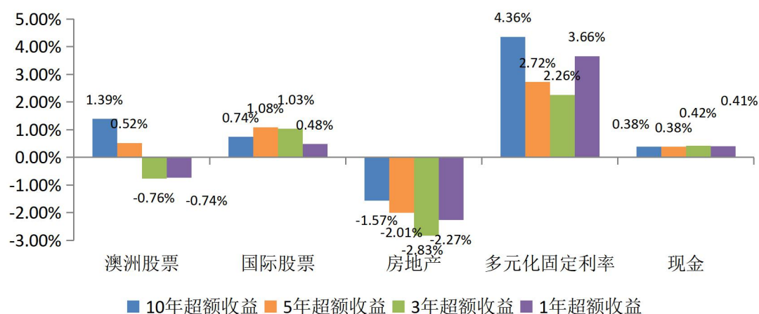
图4 CI账户各资产超额收益
