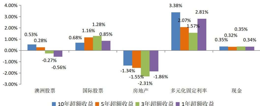
图 6 super/TTR 账户各组合超额收益
