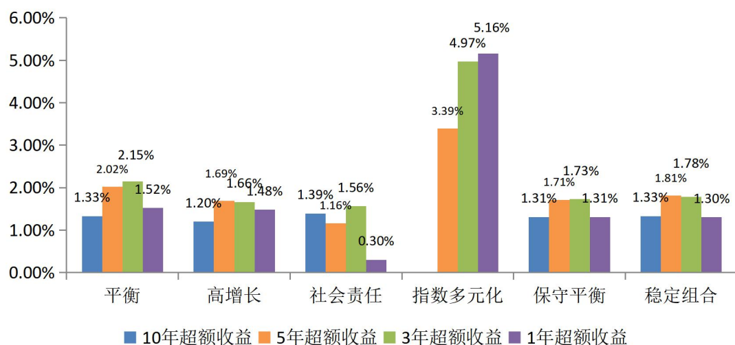
图3 CI账户各组合超额收益
